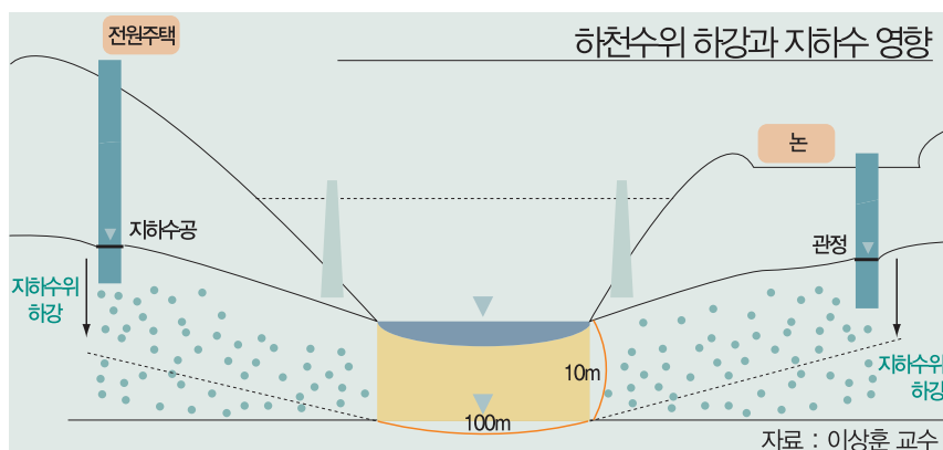
<그림 2> 홍수를 막으려고 독을 높이면 주변 지류 수위도 높아지고, 바닥을 파면 지하수가 말라버린다
